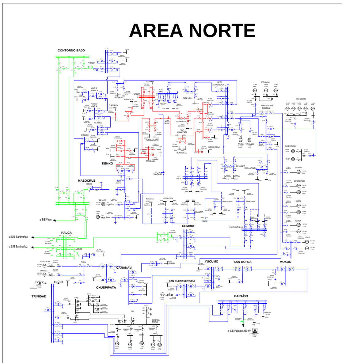
Figura 1. Diagrama unifilar SIN, área Norte
