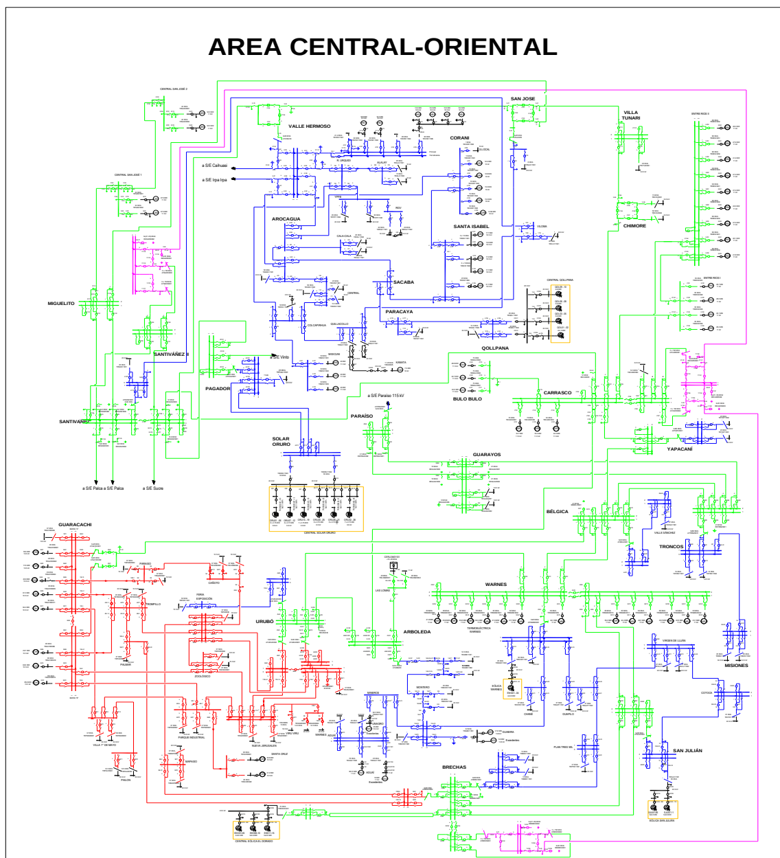
Figura 2. Diagrama unifilar SIN, área Central – Oriental
