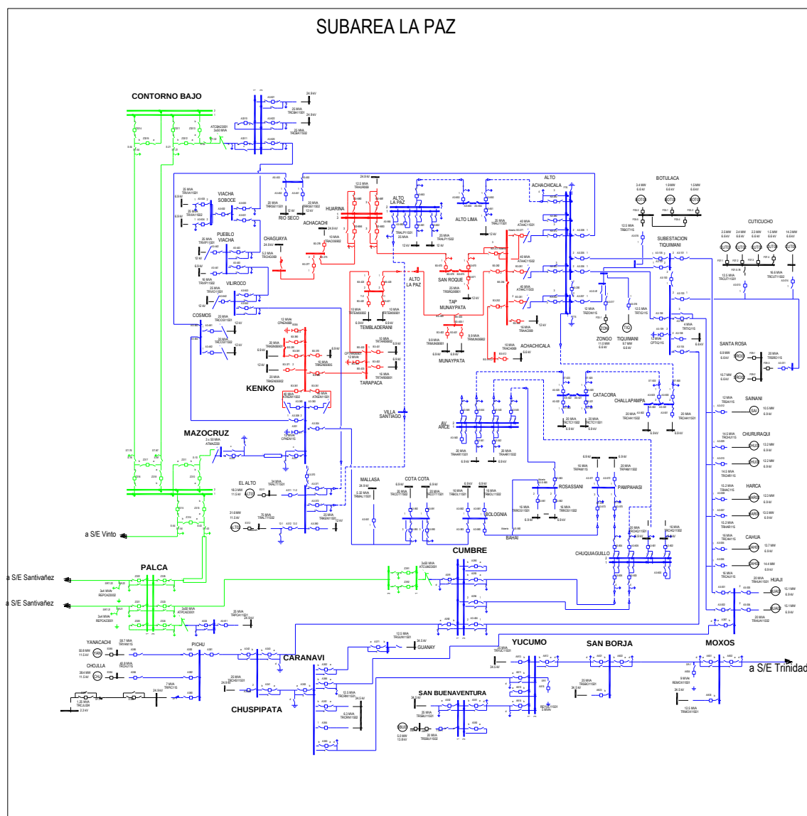
Figura 1-a. Subárea La Paz
