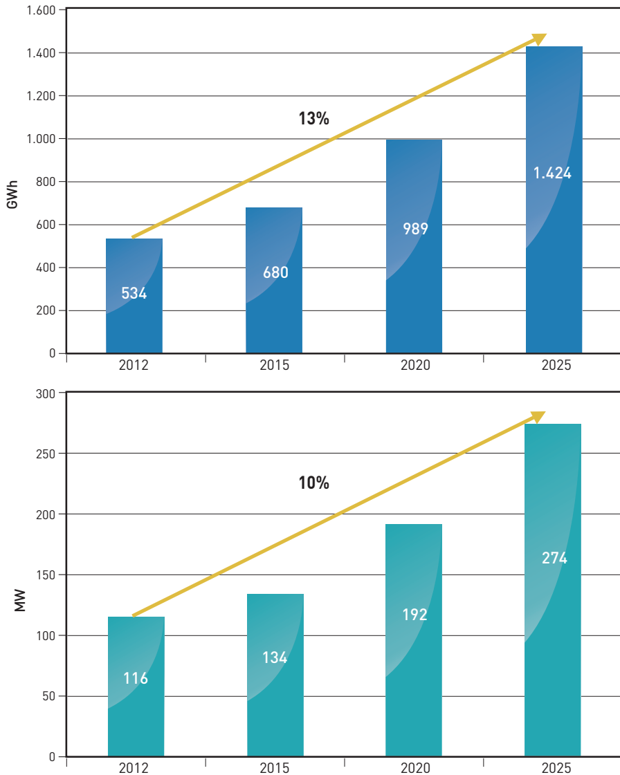
Gráfico 13 Proyección de energía y potencia al 2025 de Sistemas Aislados
